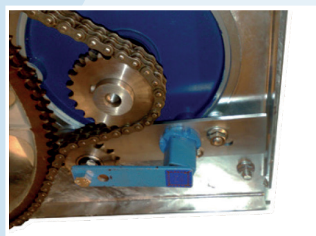
Allround 250 med automatisk kedjesträckning.
